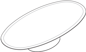
Elliptical tables, composed of n.1 table top (Q MW 360 180 S) and n.1 leg (QR 135 090) 180×180×H73 cm Q WM 360 180 S ..
