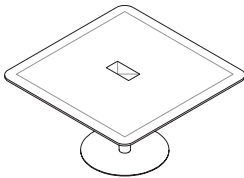
Squared tables composed of n.1 table top (Q MW 140 Q W), n.1 leg (QR 070 R W), n.1 flip access door (P DP CAB Z31) 140×140×H73 cm Q WM 140 Q W ..
