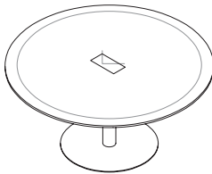
Round tables composed of n.1 table top (Q MW 160 R W), n.1 leg (QR 075 R W), n.1 flip access door (P DP CAB Z31) 160×160×H73 cm Q WM 160 R W ..
