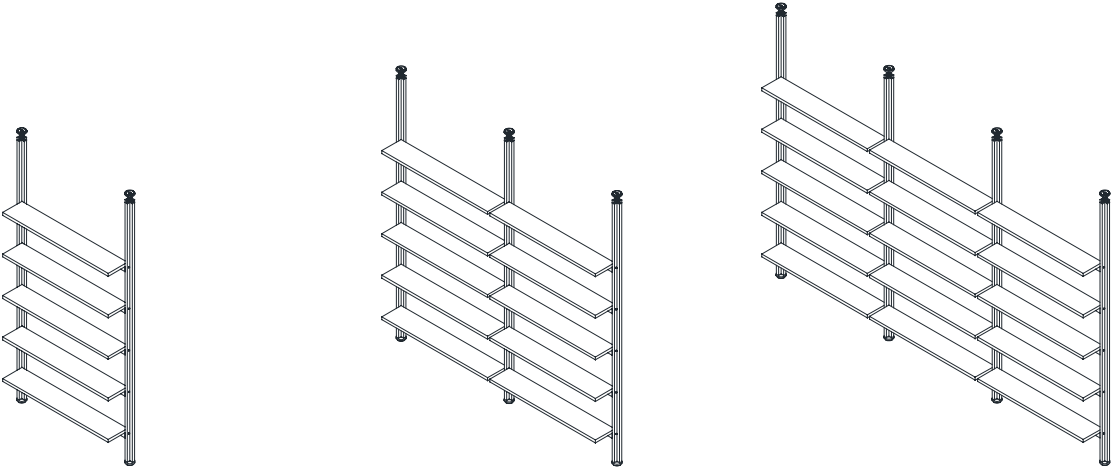
Libreria elettrificata monofacciale H. 240/269 cm con 5 mensole - 1 modulo con 2 montanti
