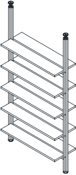
Libreria elettrificata bifacciale H. 240/269 cm con 6 mensole - 1 modulo con 2 montanti
