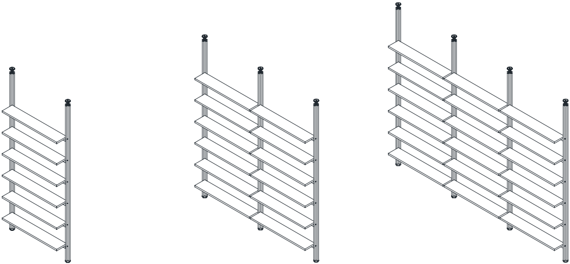
Libreria elettrificata H. 270/300 cm con 6 mensole - 1 modulo con 2 montanti
